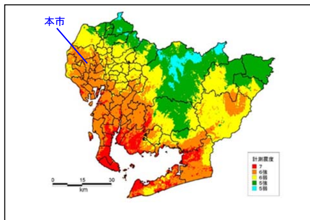
図 震度分布（陸側ケース）
